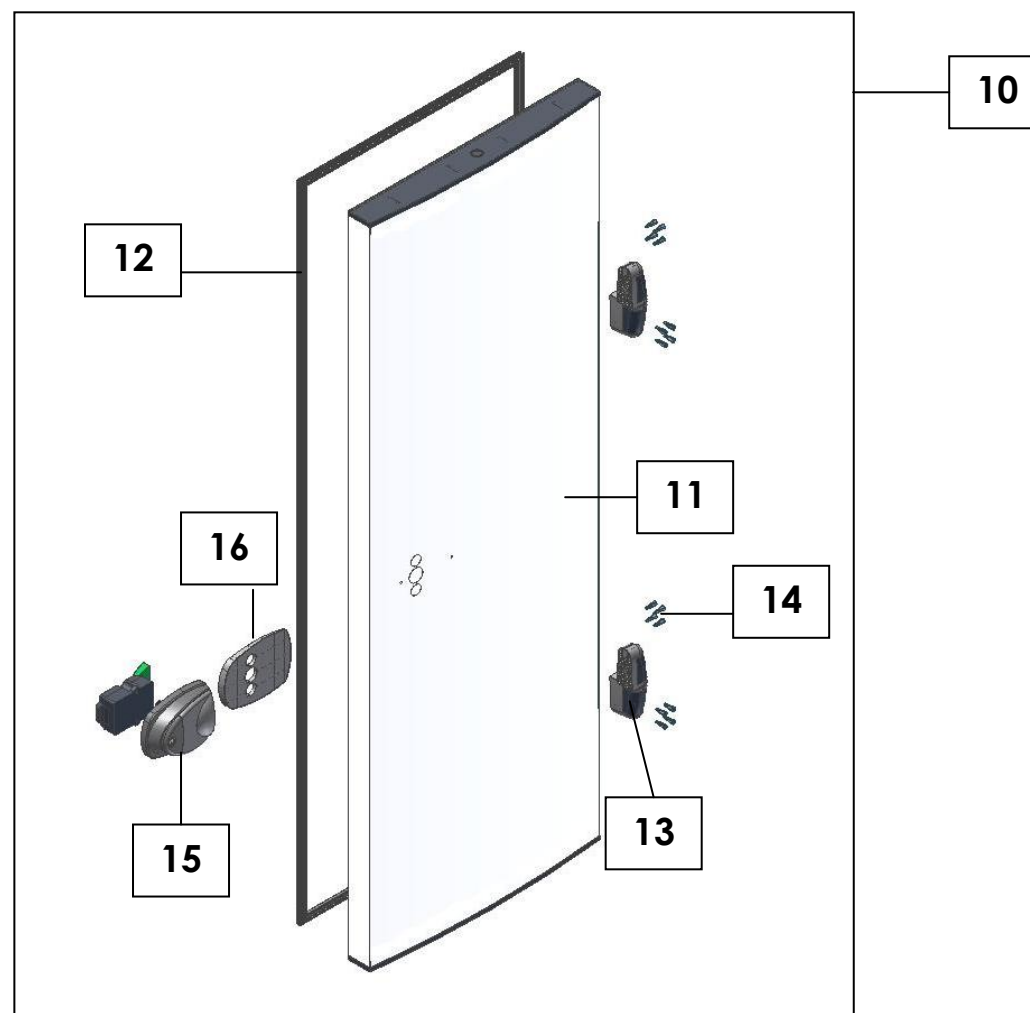
PANEL OF THE FRAME AND DOOR/ PANNEAU DU CERCEAU ET LA PORTE/WAND DES RAHMENS UND DER TÜR
