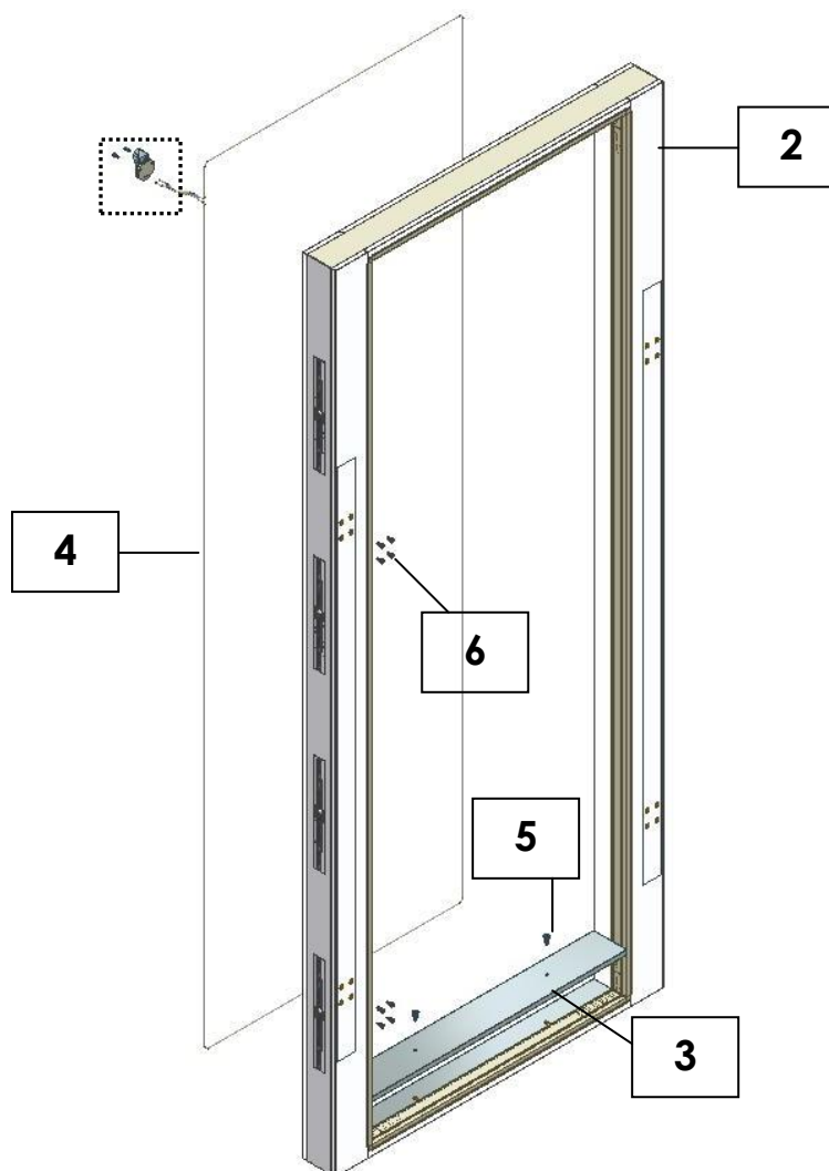
PANEL OF THE FRAME AND DOOR/ PANNEAU DU CERCEAU ET LA PORTE/WAND DES RAHMENS UND DER TÜR
