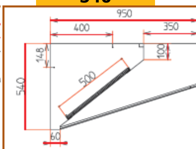
Type HR(L) 540
