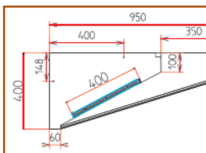
Type HR(L) 400
