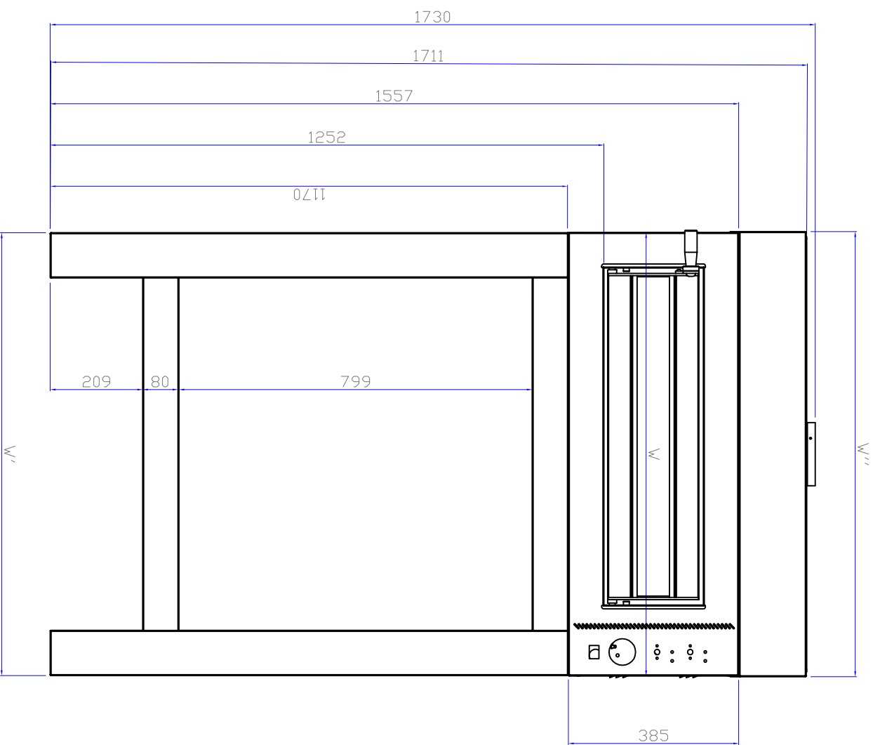
VISTA FRONTALE
