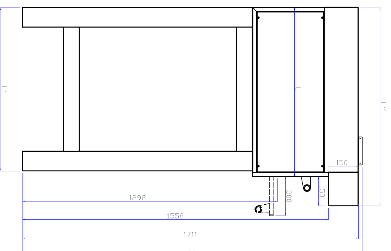
VISTA LATERALE
