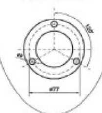
PARTICOLARE PIEDE FOOT DETAIL
